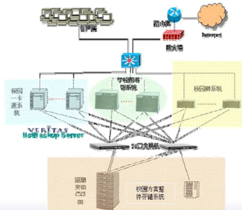
浪潮-河南工业大学项目拓扑图
